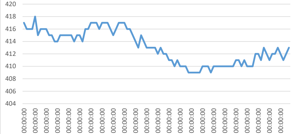
CO2
