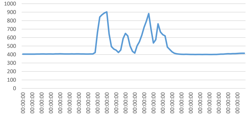
CO2
